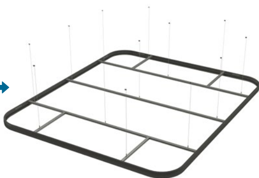
3. Fixez les profilés du cadre aux armatures et fermez le cadre.*
